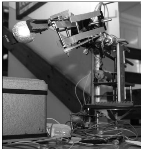
A házigazda I. Béla iskola Hadúr András, Kovács Ádám, Forray Gábor alkotta triója egy robotkart épített a versenyre
