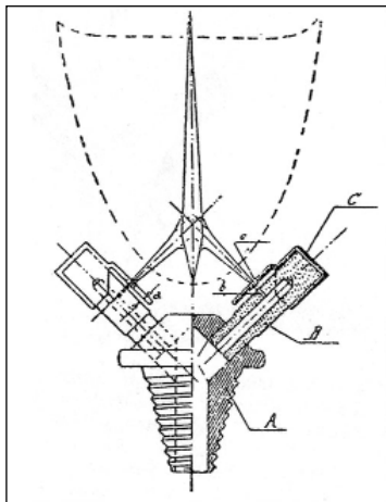
Az acetilénégő elve ...
